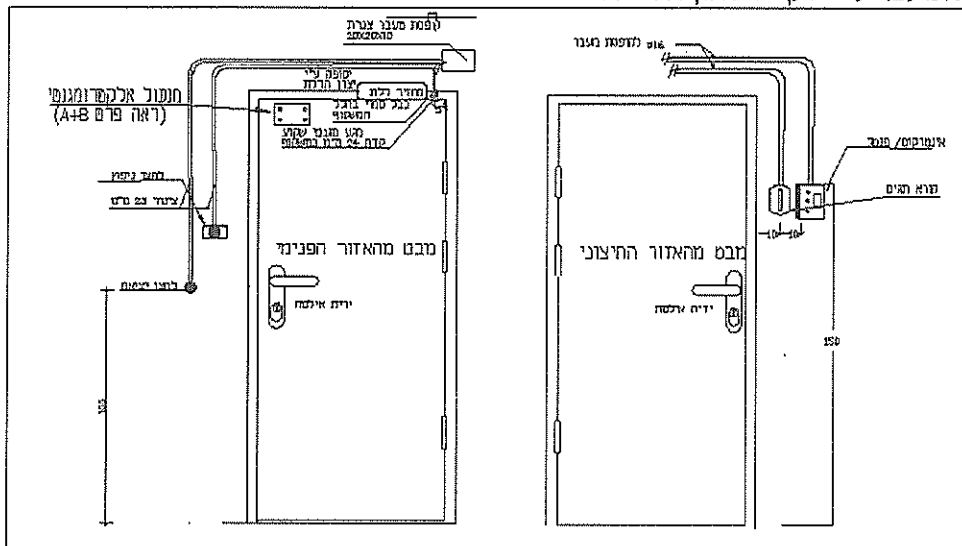
סקיצה: דלת מבוקרת אלקטרומגנטי
