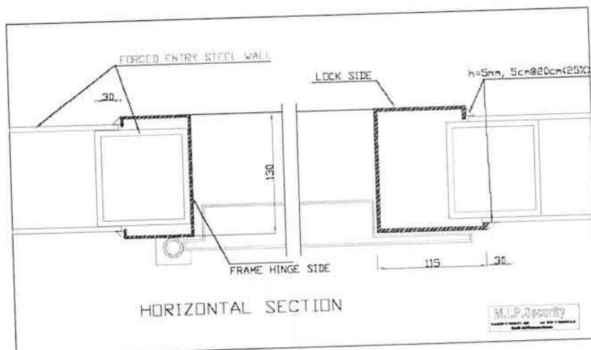
שילוב דלת או פתח מזוגג אל קיר מחופה
