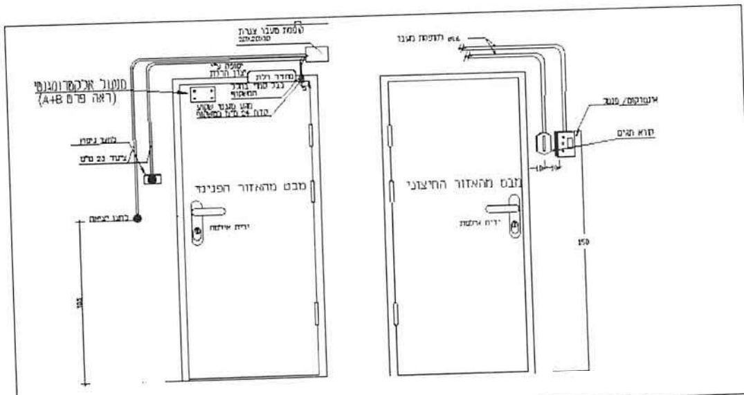
סקיצה: דלת מבוקרת אלקטרומוגנטי
