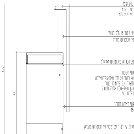
המקף במזשטח מתחרתים קליינטים 1:10
