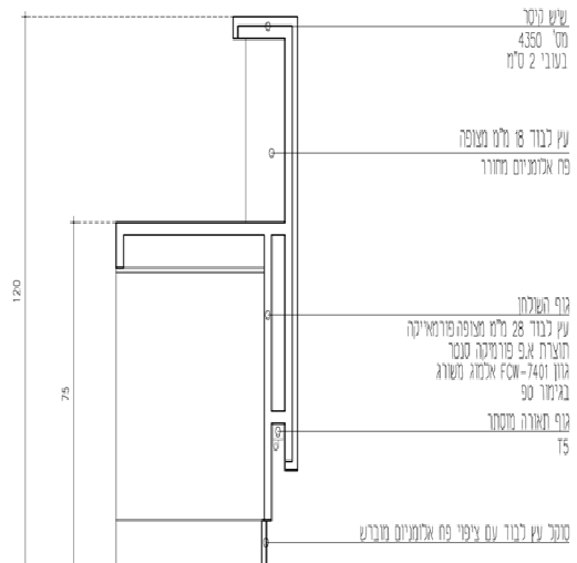
המקף במזשטח ראשי קליינטים 1:10
