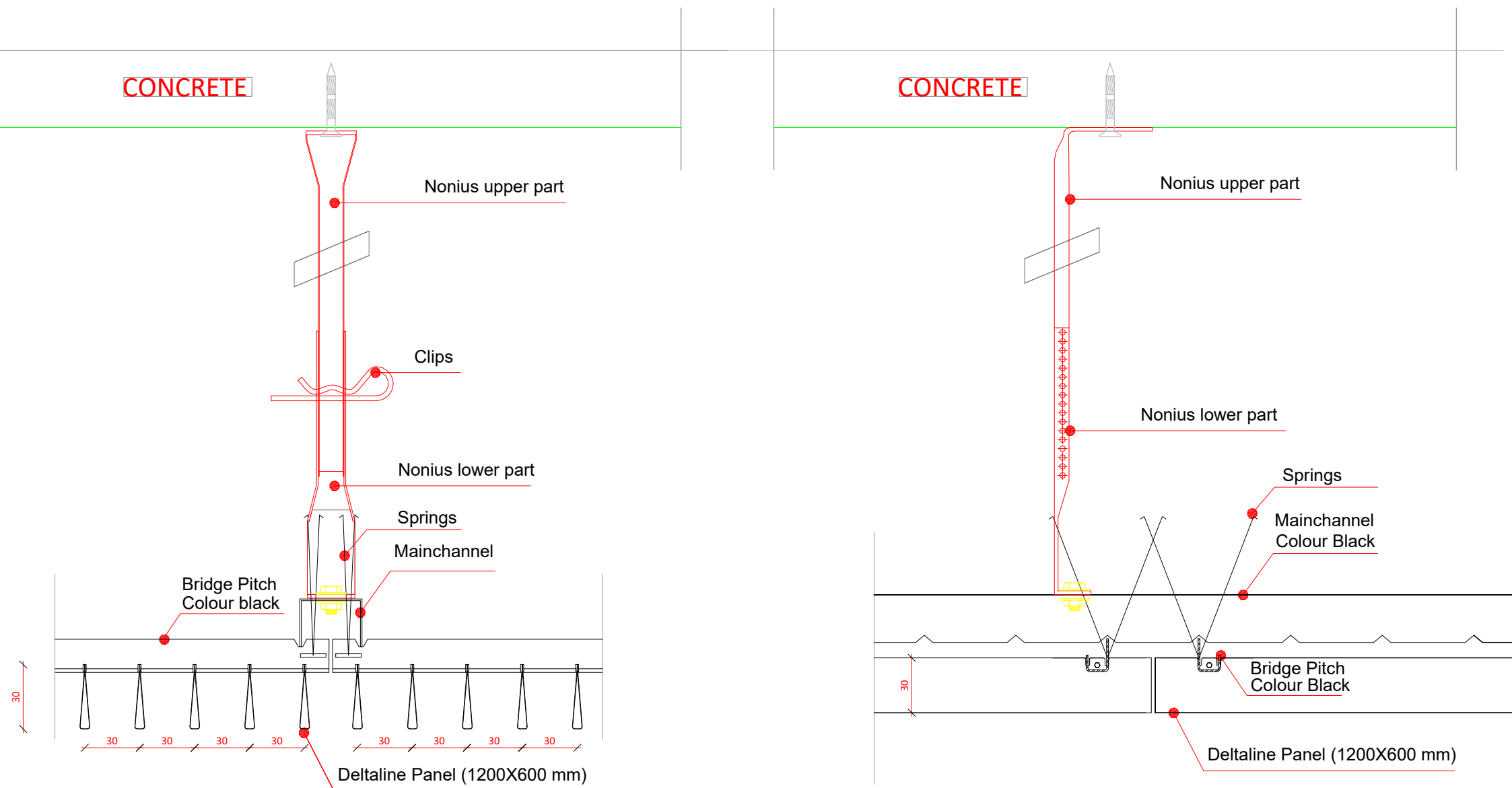
פרט תיקרה מונמכת דגם: Delta Line
