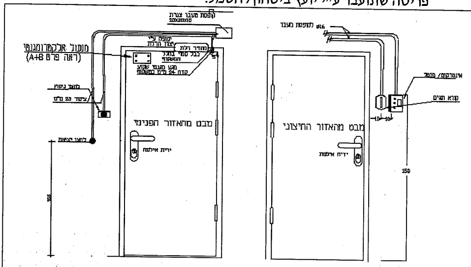
סקיצה: דלת מבוקרת אלקטרומגנטית
